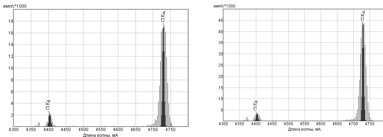
Рис. 3. Рентгенофлюорограмма коксового остатка ПВХ-пластиката (а) и ПВХ-пластиката, модифицированного органоглиной и полифосфатом аммония (б) на содержание хлора
