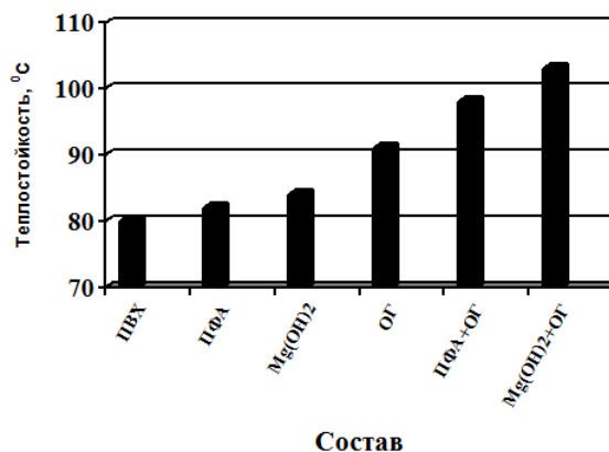
Рис. 2. Зависимость теплостойкости модифицированного ПВХ-пластиката от состава и содержания антипиренов: 1 – ПФА; 2 – Mg(OH)_2 ; 3 – ОГ; 4 – ПФА+ОГ; 5 – Mg(OH)_2 +ОГ
