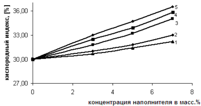
Рис. 1. Зависимость кислородного индекса ПВХ-пластиката от состава и содержания антипиренов: 1 – ПФА; 2 – Mg(OH)_2 ; 3 – ОГ; 4 – ПФА+ОГ; 5 – Mg(OH)_2 +ОГ
