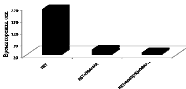
Рис. 2. Зависимость времени горения композитного ПБТ от состава наполнителя
